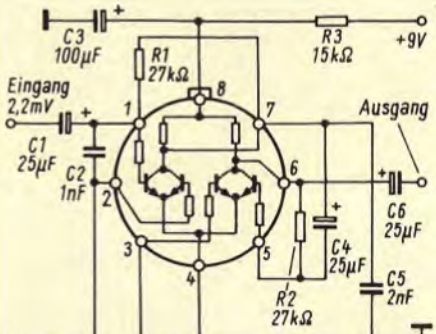
Bild 3b. Zweistufiger Wechselspannungsverstärker
