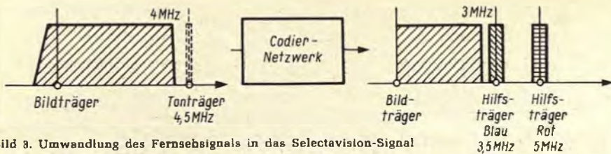
Bild 3. Umwandlung des Fernsehsignals in das Selectavision-Signal
