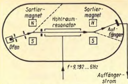
Bild 2. Prinzip des CS-Resonators
