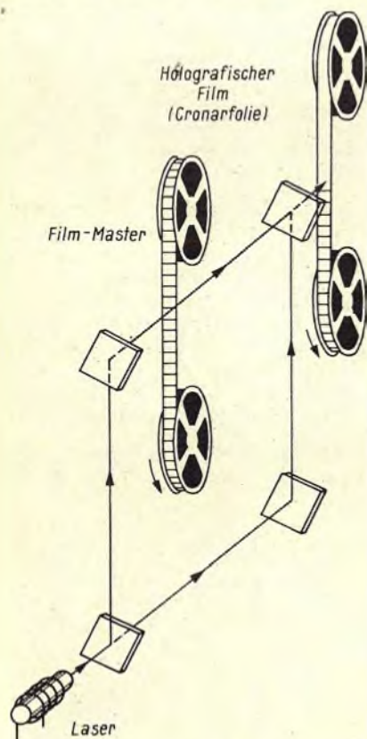
Bild 4. Herstellung des Hologramm-Masters aus dem Film-Master
