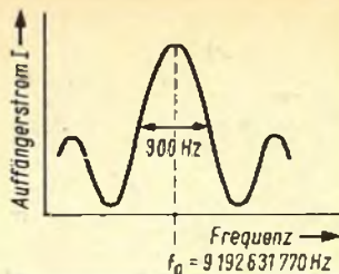
Bild 3. Resonanzkurve des CS-Resonators
