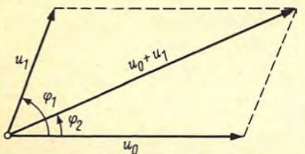
Bild 8b. Vektorielle Addition. Pfeillänge = Amplitude der Sinusspannung, \varphi_1 und \varphi_2 = Phasenwinkel zur Bezugsspannung u_0
