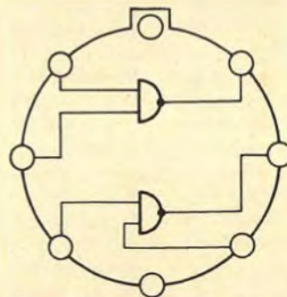
Bild 1a. Der Baustein RTL 914 von SGS mit der in der logischen Schaltungstechnik üblichen Darstellungsart
