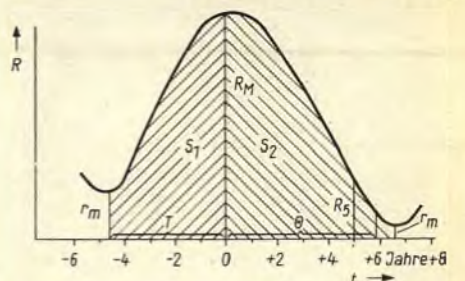
Bild 10. Schematische Darstellung eines Sonnenfleckenzyklus
