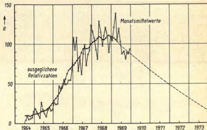
Bild 2. Sonnenfleckenzyklus Nr. 20
