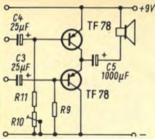
Bild 6. Gegentakt-Endstufe mit pnp-Transistoren
