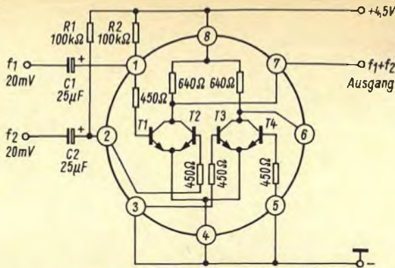
Bild 7b. Schwebung durch Mischung von f_1 und f_2
