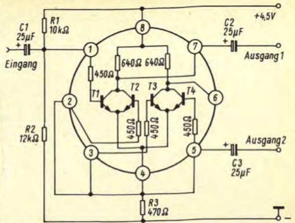
Bild 4a. Einstufiger Phasenaufsplitter
