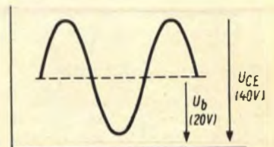
Rechts: Bild 3. Verhältnis von Speisespannung zur zulässigen Kollektoremitter-Spannung in einer Gegentakt-Endstufe
