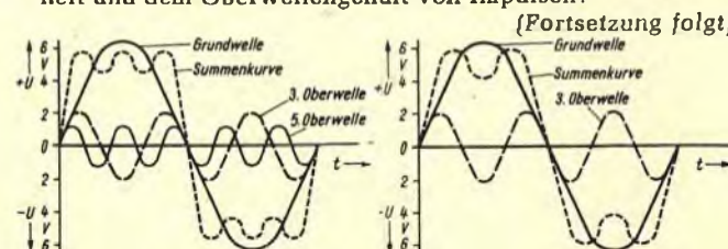
Bild 2.9. Aufbau von Rechteckwechselfspannungen aus Oberwellen
