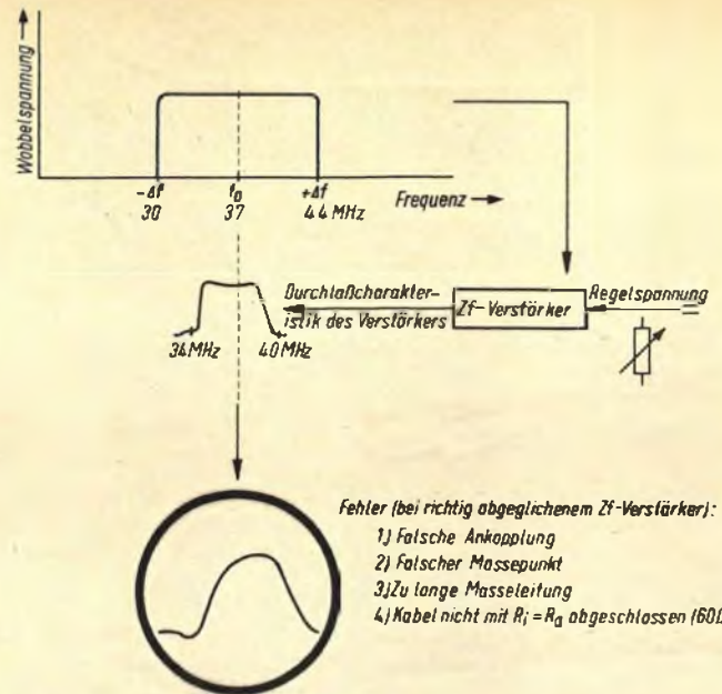
Bild 55. Falsche Durchlaßkurve durch Fehlanpassung des Wobblers
