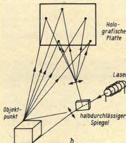
Bild 1. Während der Objekt-punkt bei der fotografischen Aufnahme (a) nur eine Stelle der lichtempfindlichen Filmschicht schwärzt, ist im Hologramm (b) der Objekt-punkt in jeder Stelle des Interferenzbildes enthalten
