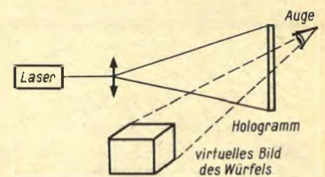
Bild 2. Rückgewinnung des dreidimensionalen virtuellen Bildes aus dem mit kohärentem Licht durchleuchteten Hologramm
