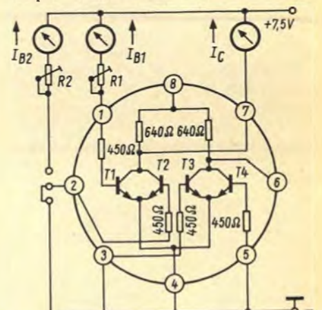
Bild 2. Prüfschaltung zum Aufnehmen der wichtigsten Kenndaten
