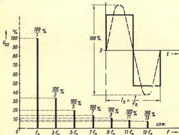
Bild 2.8. Frequenzen und Amplituden der Oberwellen einer Rechteckwechselfspannung
