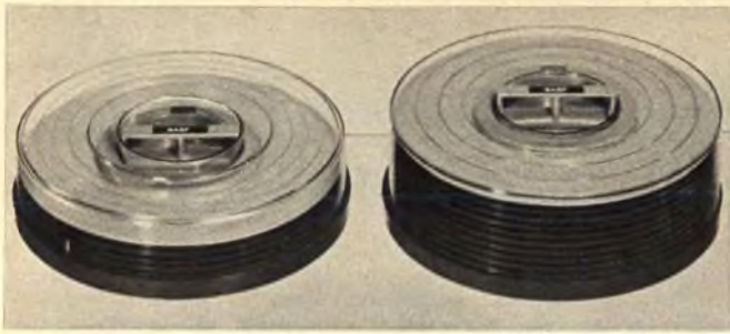
Magnetplattenstapel der BASF. Links Typ 618, auf dessen sieben nutzbaren Plattenseiten mehr als sieben Millionen Informationen festgehalten werden können; rechts: Typ 621 mit zwanzig nutzbaren Plattenseiten
