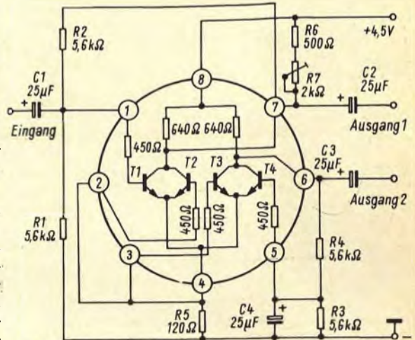
Bild 4b. Zweistufiger Phasenaufsplitter
