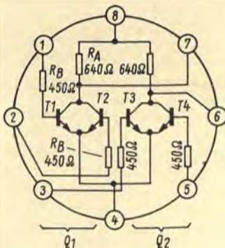
Bild 1b. Innenaufbau der integrierten Schaltung (Realschaltung)
