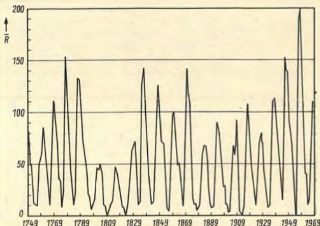
Bild 1. Sonnenfleckenzyklen von 1749 bis 1969
