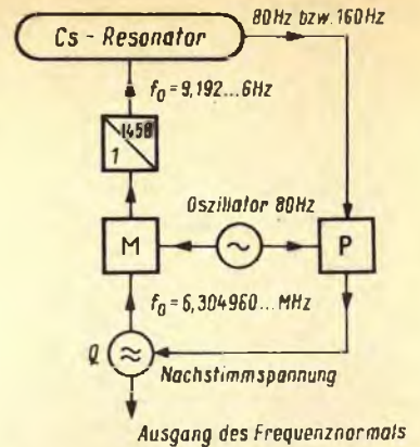
Rechts: Bild 4. Vereinfachtes Blockschaubild eines absoluten Frequenznormals
